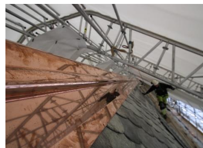
1, Mønebeslaget mangler kun loddingene før takpresenningen blir tatt bort og mønespiret blir montert.
