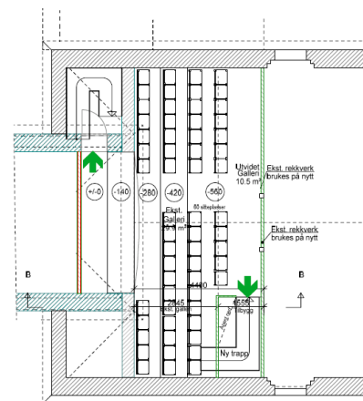
Plan 2. etasje galleri 80 sitteplasser
