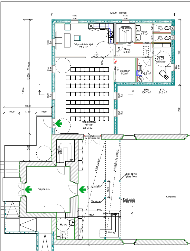
Plan 1. etasje m/tilbygg menighetssal
