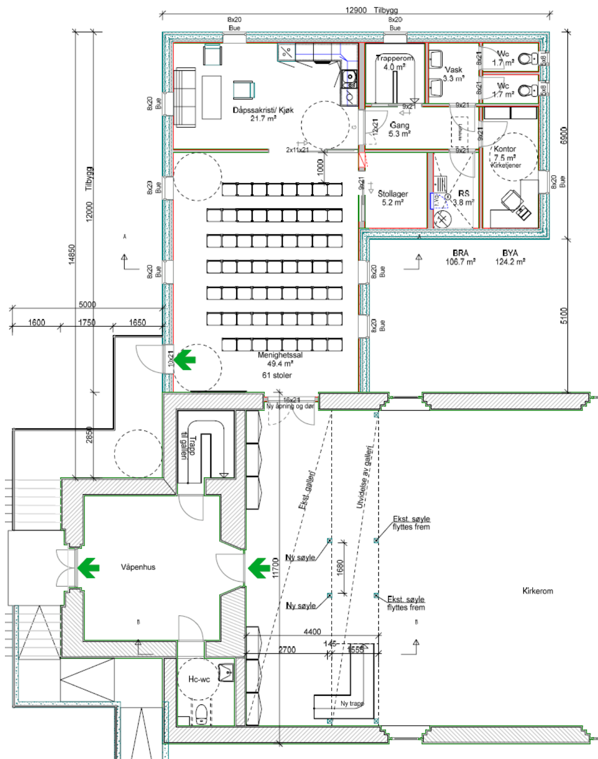
Plan 1. etasje m/tilbygg menighetssal
