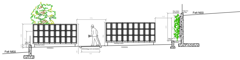
SNITT B-BB
