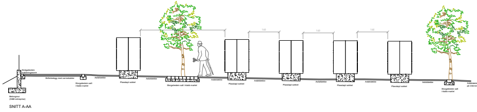
SNITT A-AA
