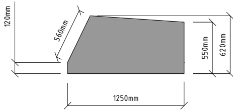
Profil fundament
