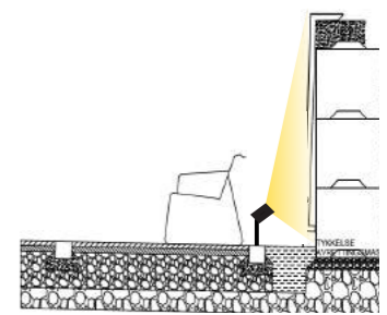
Snitt pullert: avskjermnet spot plassert bak sittebenk på jordspyd.
