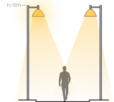
Snitt mast/gangvei: 5m høy mast med opal skjerm og god avblending, asymmetrisk optikk.
