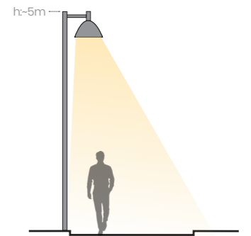
Snitt mast/gangvei: 5m høy mast med god avblending og asymmetrisk optikk med direkte lys ned på gangareal.
