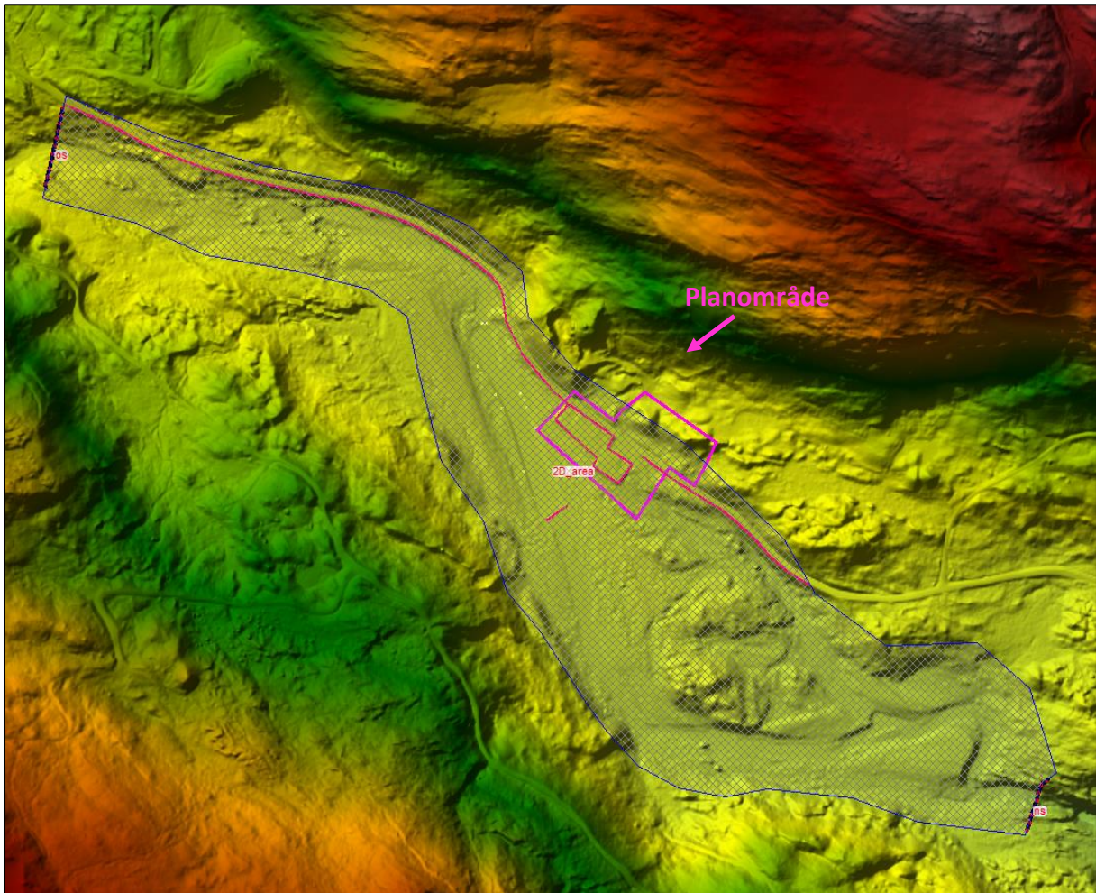
Figur 10: Benyttet terrengmodell, beregningsgrid og plassering av grensebetingelser.
