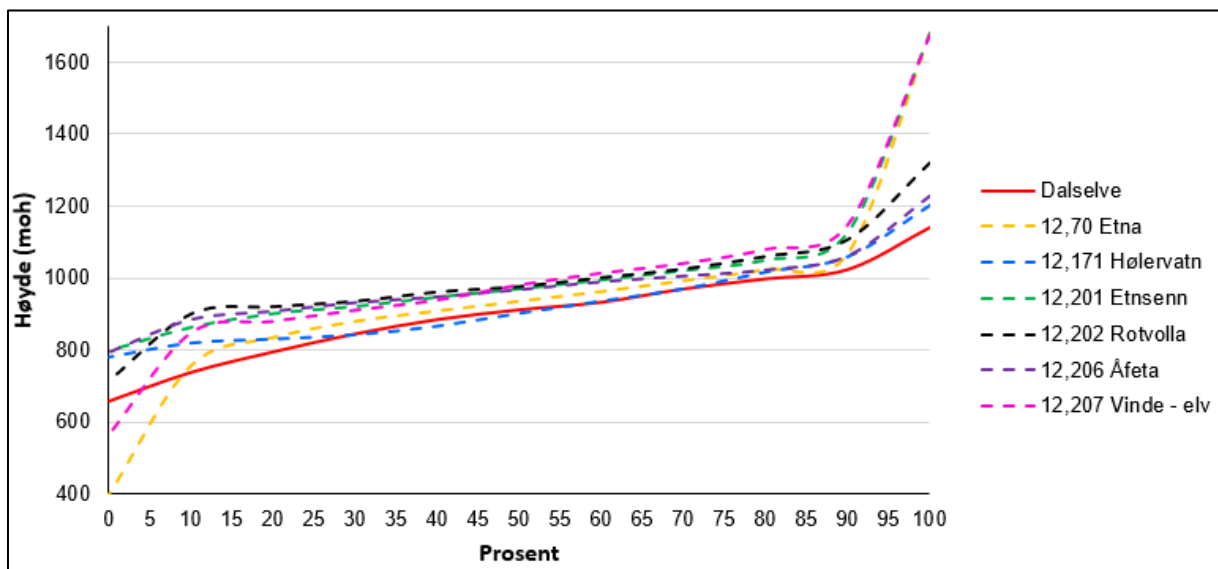
Figur 8: Hypsografisk kurve for Dalselve og utvalgte referansefelt.
