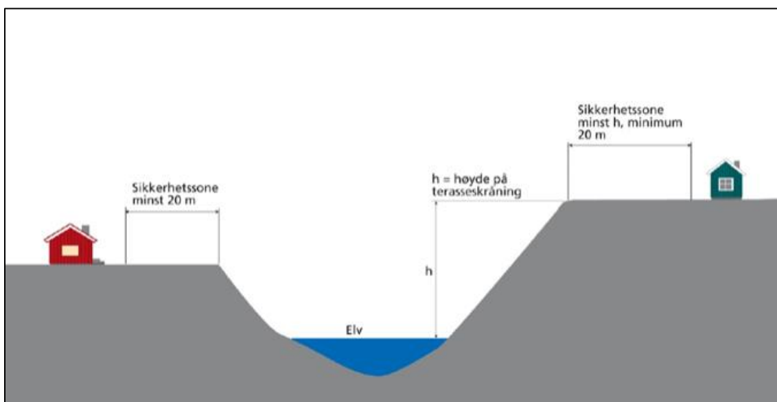
Figur 13: Sikkerhetssone mot erosjon (DiBK, 2016).
