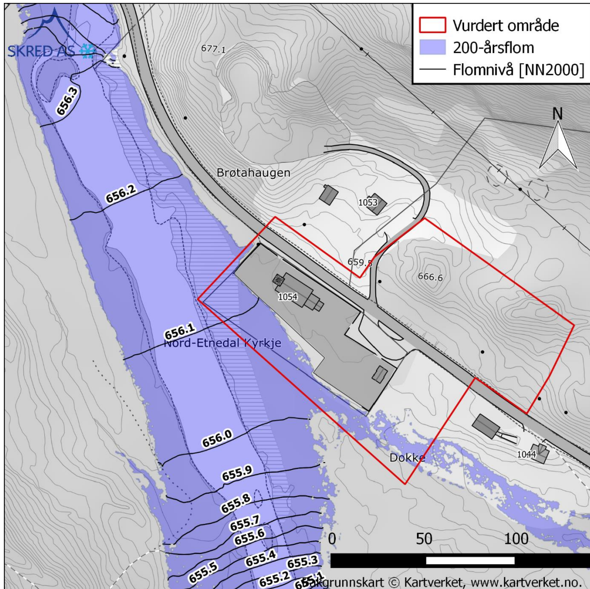
Figur 12: Estimert 200-års flomsone og flomnivåer for Dalselve ved Nord-Etnedal kirke.
