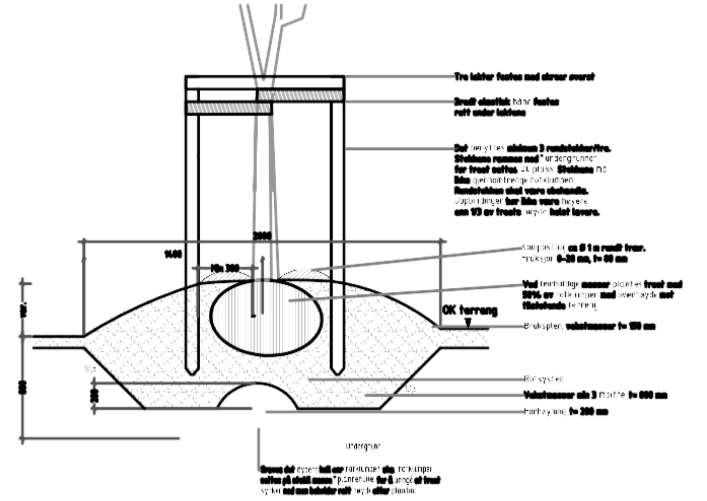
PRINSIPP TREPLANTING PÅ LEIRHOLDIG JORD M 1:20
