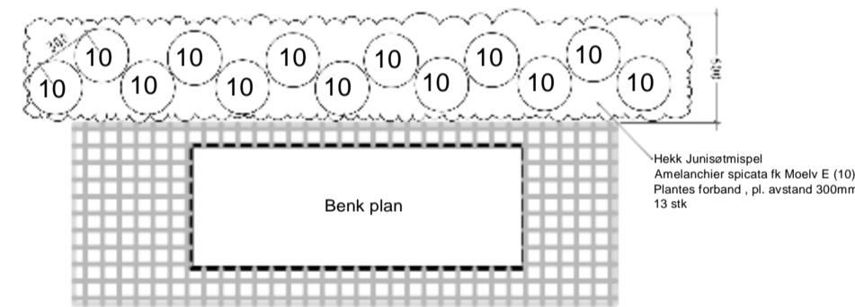
PLANTEPRINSIPP A- BENK MED HEKK - M 1:25
