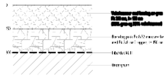
PRINSIPPSNITT OPPBYGNING GRUSFORSTERKET GRESS M 1:10
