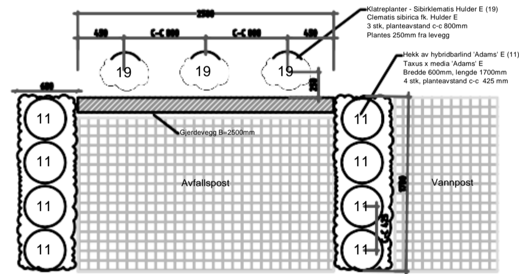
PLANTEPRINSIPP B - AVFALLSTASJON - M 1:25
