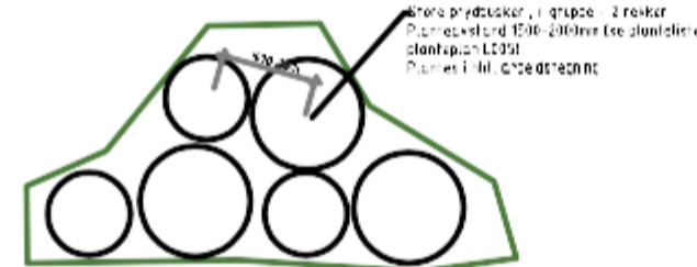
PLANTEPRINSIPP C C2- FRI BUSKBEPLANTNING DOBBEL REKKE M 1:100
