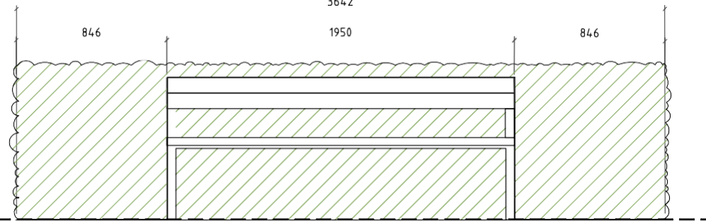
GJERDEVEGG AVFALLSPOST OPPRISS M1:20
