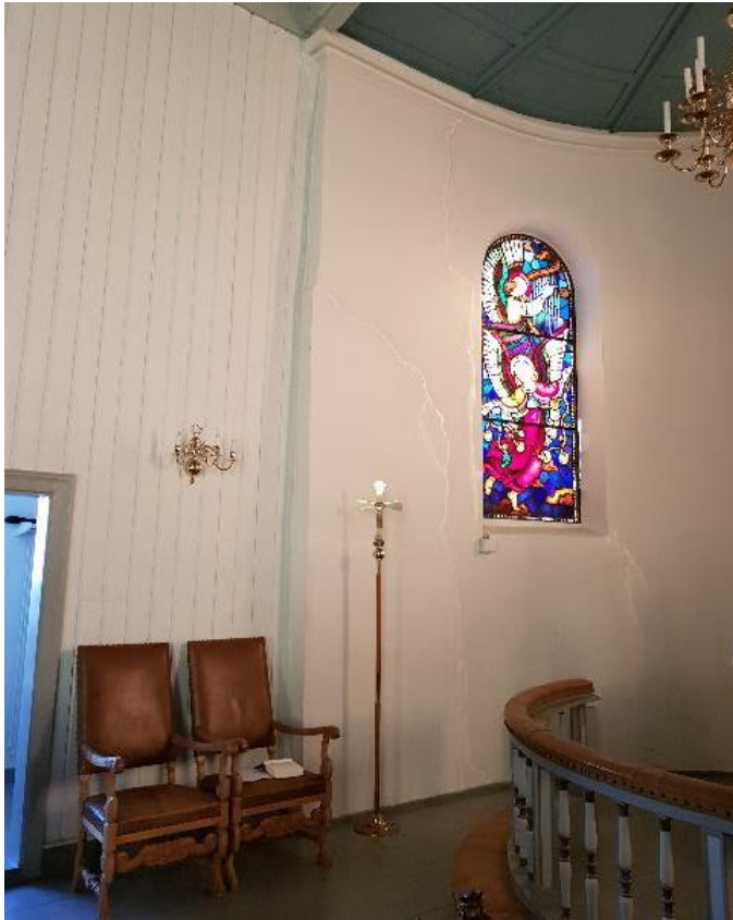
Fig17: Sprekker på nordvegg i apsis
