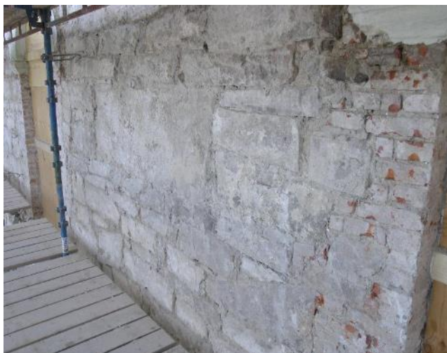
Fig.3: Sørfasaden etter at pussen var hugget i 2010.
