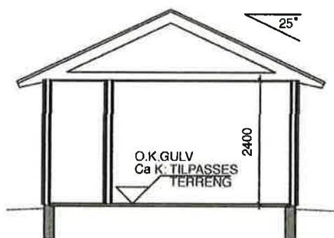
SNITT B-B
