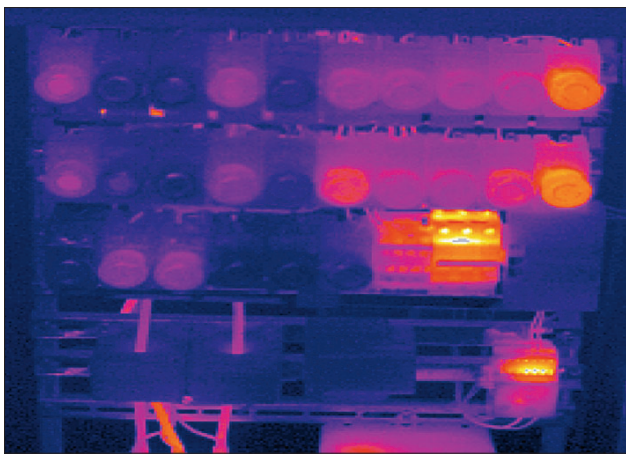
Termografi frå 2006 av sikringsskapet i Eksingedalen viser temperaturskilnader i sikringsskapet. Ljose fargar er høg temperatur. Eit rele som var for varmt, og ein kurs som var høg belastning på, vart reparert.
